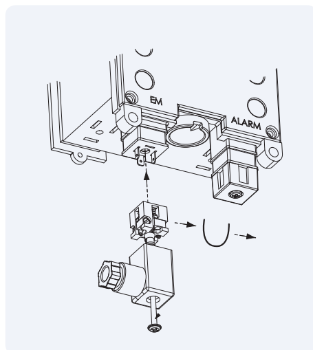
Obr. 7.6: Zapojení na přípojku řízení energie
