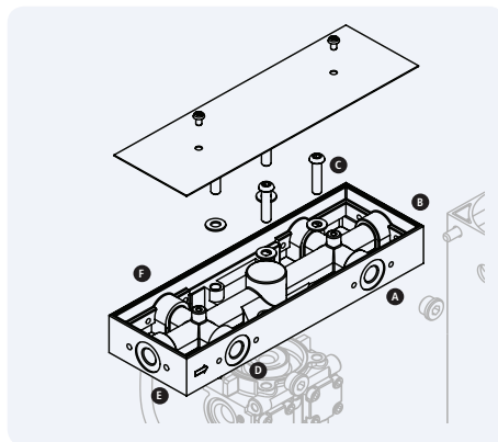
Obr. 3.6: Změna konfigurace vstupních/výstupních přípojek.
