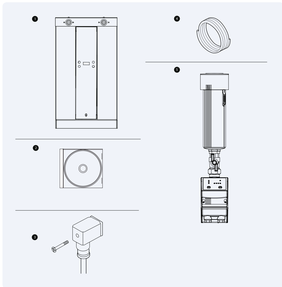
Obr. 2.1: Rozsah dodávky
