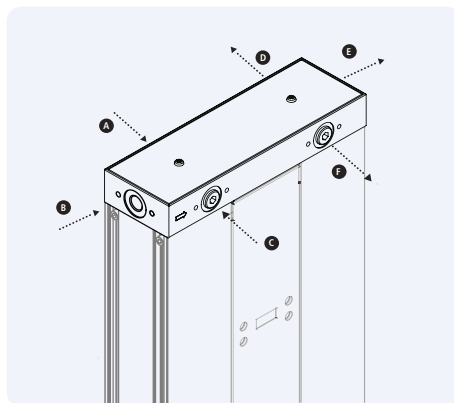
Obr. 3.5: Vstupní/výstupní přípočky
