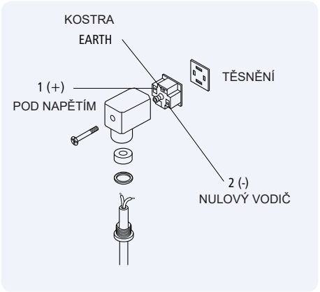
Obr. 4.1: DIN konektor
