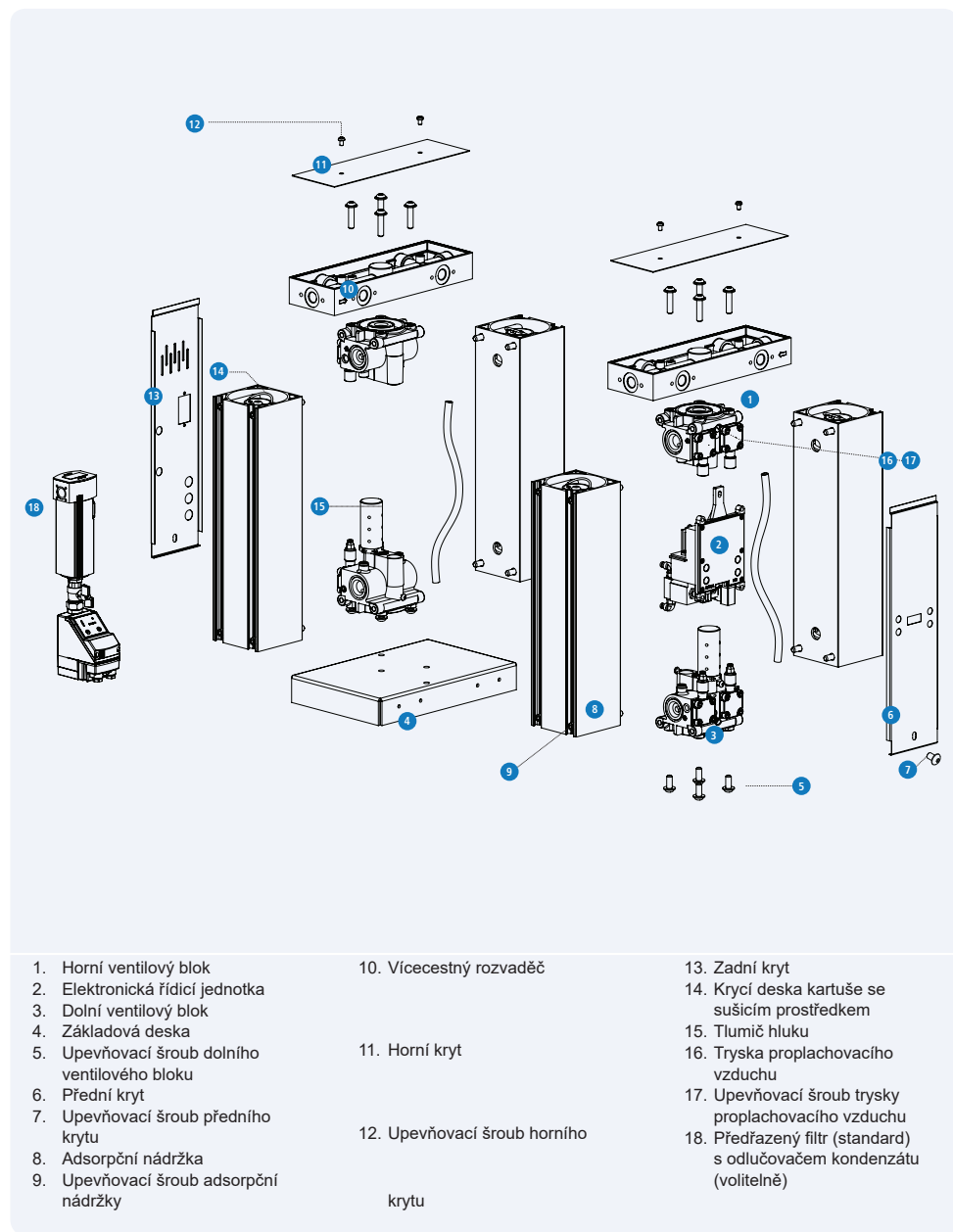
Obr 2.3 Komponenty DRYPOINT® AC 191 - 196
