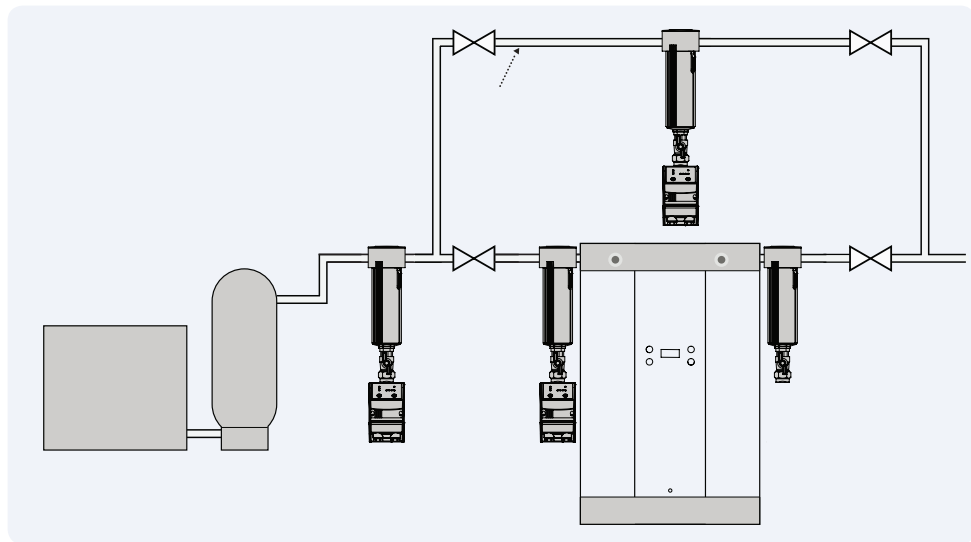
Obr. 3.13: Typická instalace
