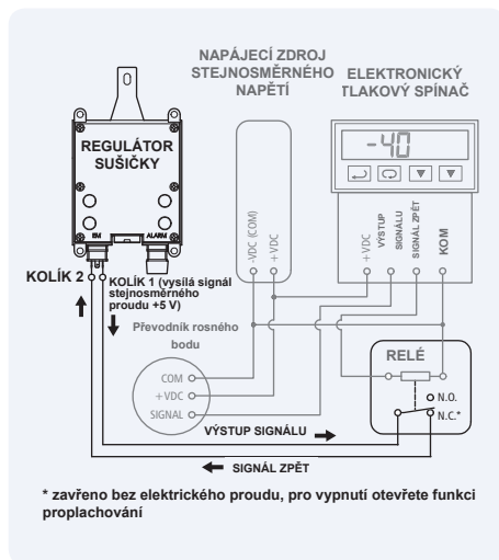
Obr. 7.5: použití procesního regulátoru
