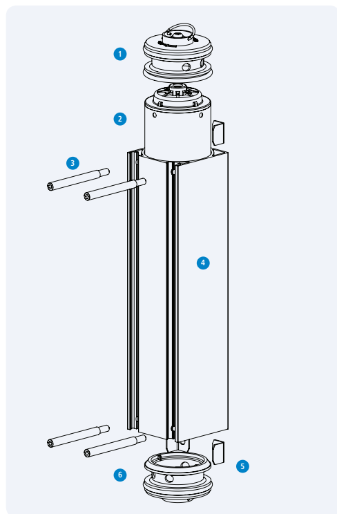
Obr. 10.5 Sestava adsorpční nádržky
