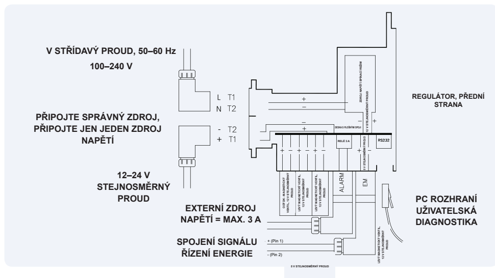
Obr. 4.3: 100 až 240 V střídavý proud
