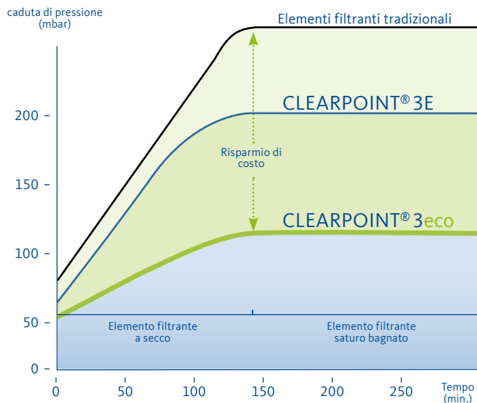
I costi di utilizzo dei filtri CLEARPOINT® 3eco sono stati sensibilmente ridotti. Il grafico mostra i filtri flangiati con grado di filtrazione S e portata dimensionata per il massimo risparmio energetico.
