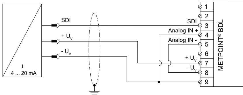
3線式 SDIインターフェースの結線図
