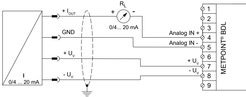
アナログ4線式 0/4 ...の結線図20 mA
