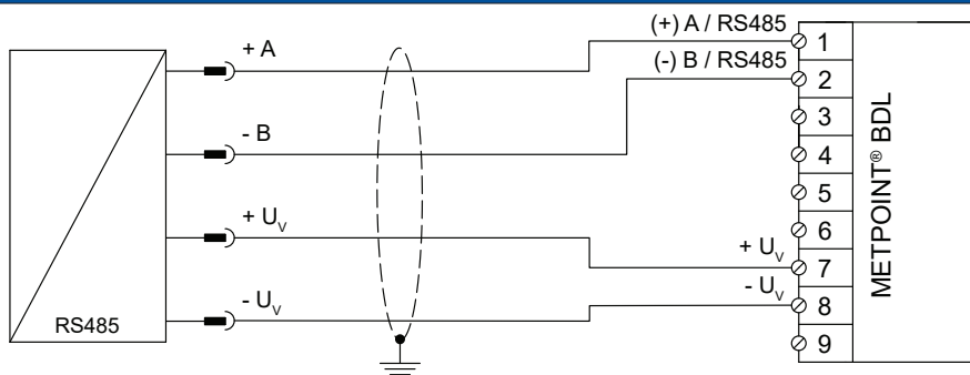
双方向バスシステム RS485の結線図
