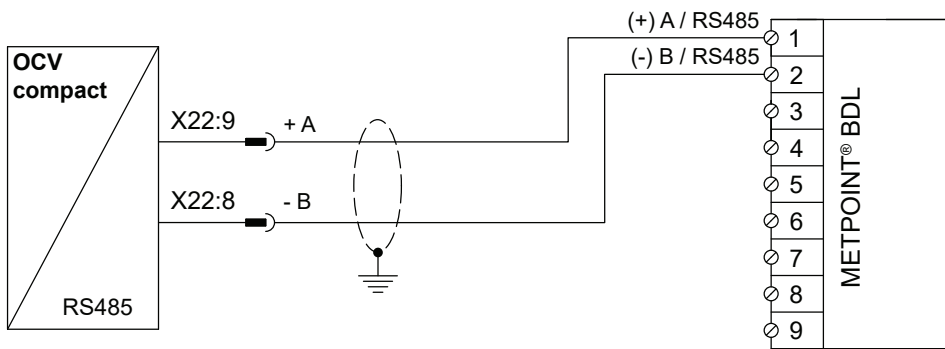
METPOINT® OCV compact 及びMETPOINT® BDLの結線図
