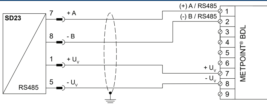
METPOINT® SD23及びMETPOINT® BDLの結線図
