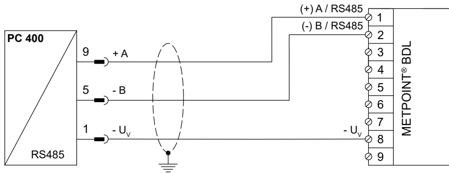
PC 400及びMETPOINT® BDLの結線図
