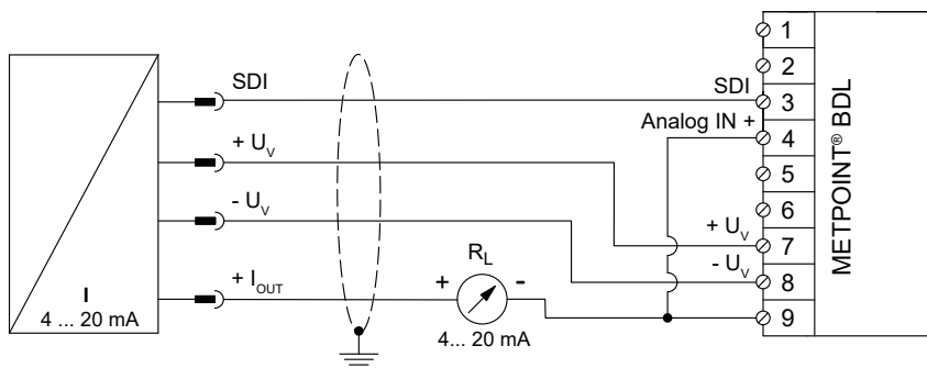
4線式 SDIインターフェースの結線図
