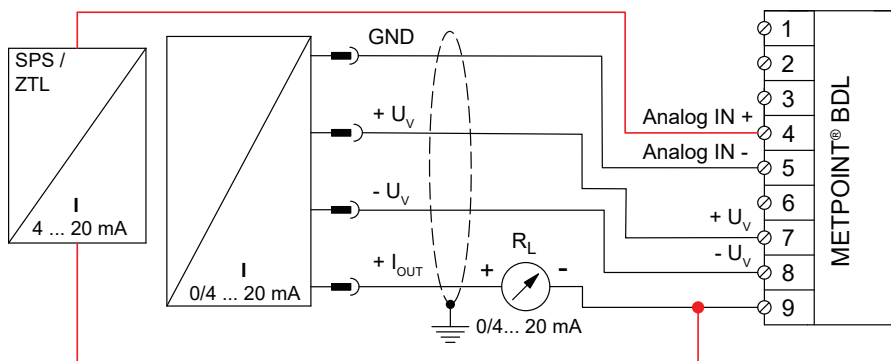
アナログ4線式 0/4 ...の結線図20 mA
