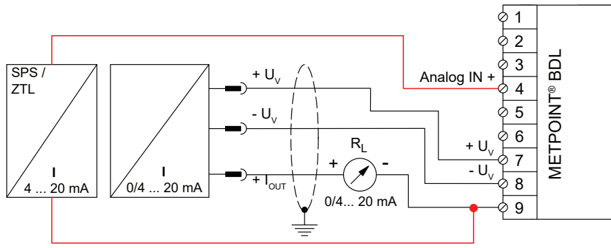
アナログ3線式 0/4 ...の結線図20 mA
