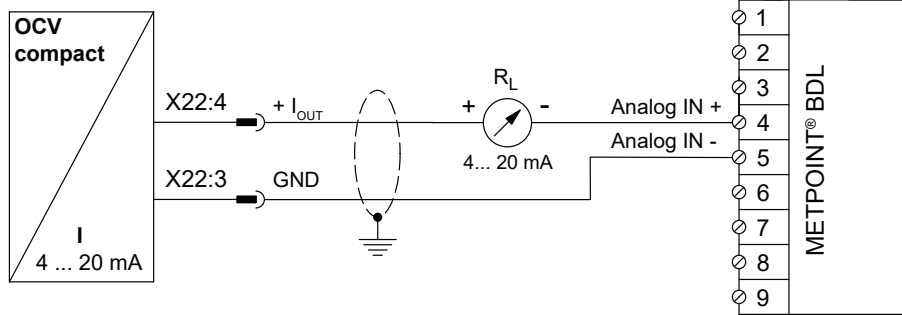
METPOINT® OCV compact 及びMETPOINT® BDLの結線図
