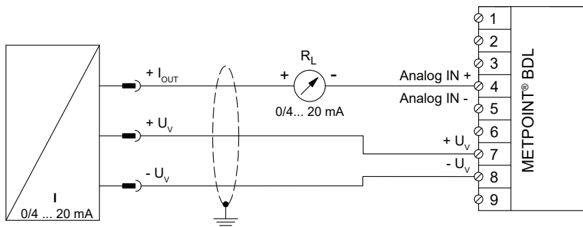
アナログ3線式 0/4 ...の結線図20 mA
