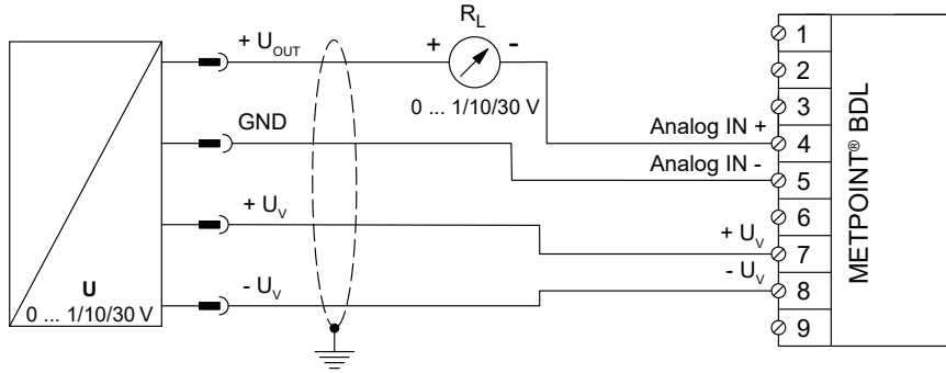
アナログ4線式 0 ...の結線図1/10/30 V
