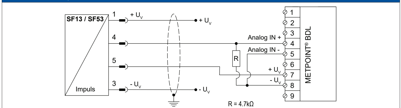
METPOINT® SF13 / SF53及びMETPOINT® BDLの結線図
