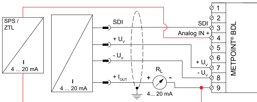
4線式 SDIインターフェースの結線図
