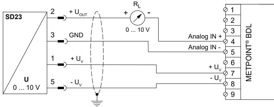
METPOINT® SD23及びMETPOINT® BDLの結線図
