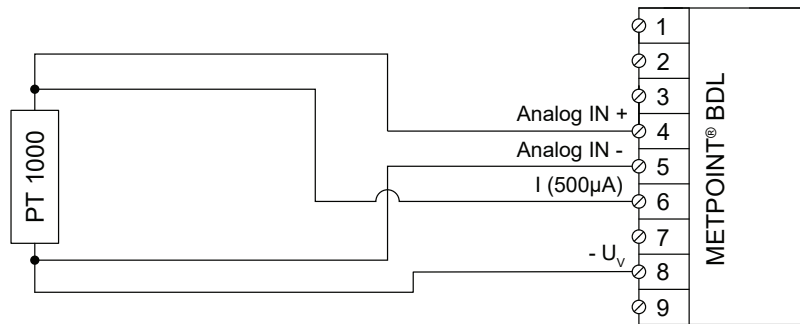
PT 1000及びMETPOINT® BDLの結線図
