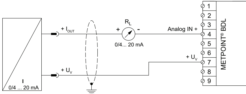
アナログ2線式 0/4 ...の結線図20 mA
