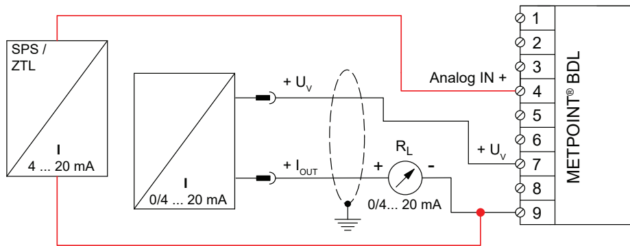
アナログ2線式 0/4 ...の結線図20 mA
