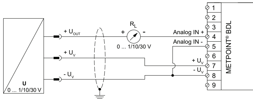
アナログ3線式 0 ...の結線図1/10/30 V
