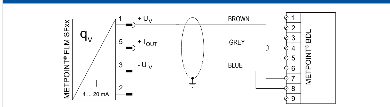
METPOINT® SF53及びMETPOINT® BDLの結線図
