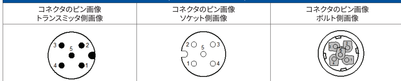
コネクタBのピンサイン、M12×1、5ピン、A符号化(EN 61076-2-101による)
