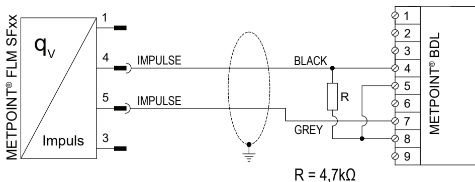
METPOINT® SF53及びMETPOINT® BDL / BDL V2の結線図
