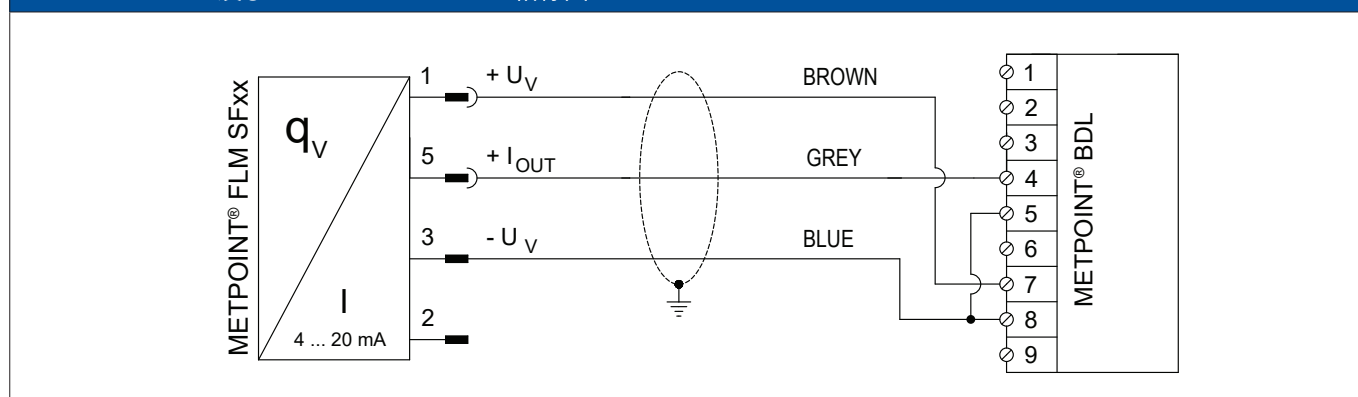
METPOINT® SF53及びMETPOINT® BDL V2の結線図
