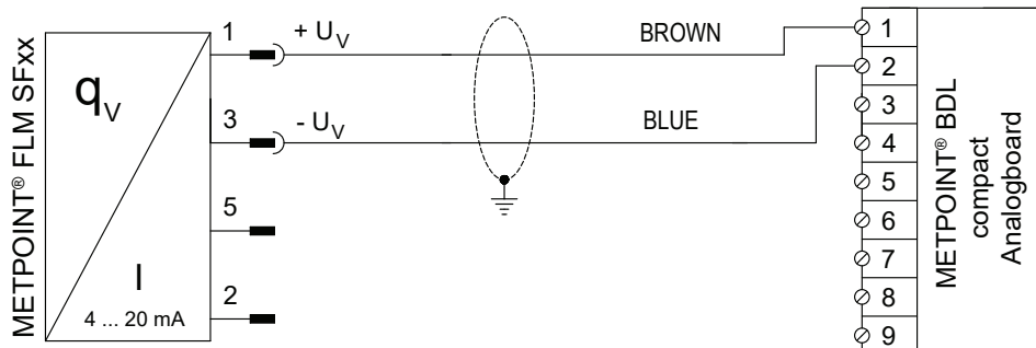
METPOINT® SF53 und METPOINT® BDL compact(アナログボード)の結線図
