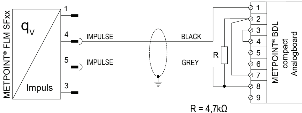
METPOINT® SF53 und METPOINT® BDL compact(アナログボード)の結線図
