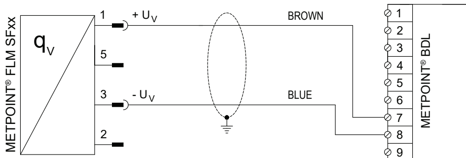
METPOINT® SF53及びMETPOINT® BDL / BDL V2の結線図
