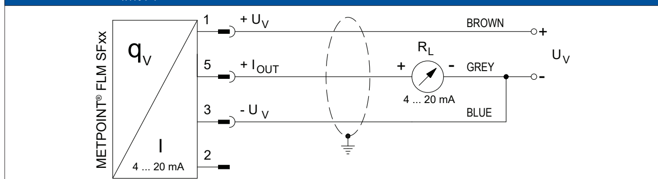
METPOINT® SF53 の結線図
