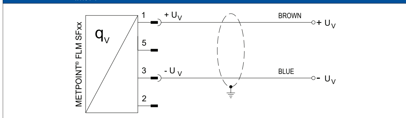
METPOINT® SF53 の結線図
